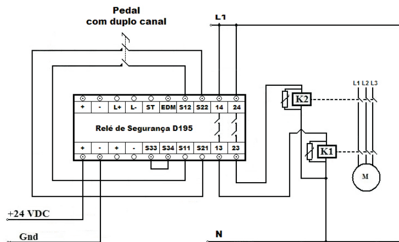
Relé de Segurança D195 com Partida por Pedal
