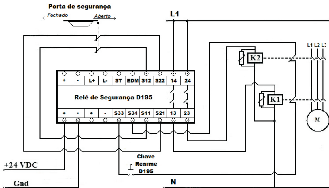
Diagrama elétrico do Relé de Segurança D195 quando utilizado como interface para uma Porta de Segurança ( Safety Gate )
