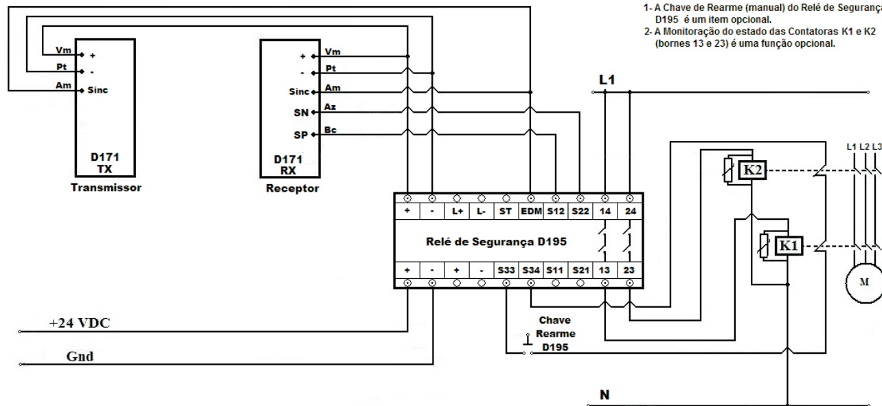
Diagrama elétrico do Relé de Segurança D195 quando utilizado como interface para o Sensor Laser D171
