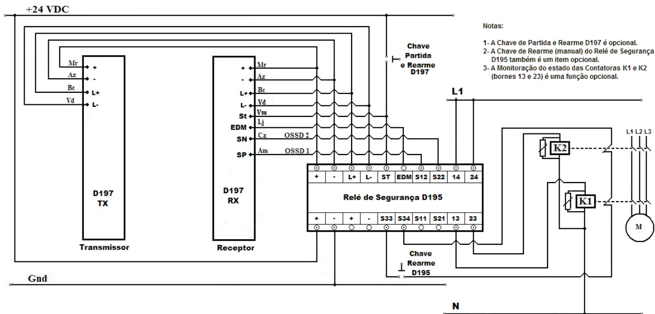
Diagrama elétrico do Relé de Segurança D195 quando utilizado como interface para a Cortina de Luz D197
