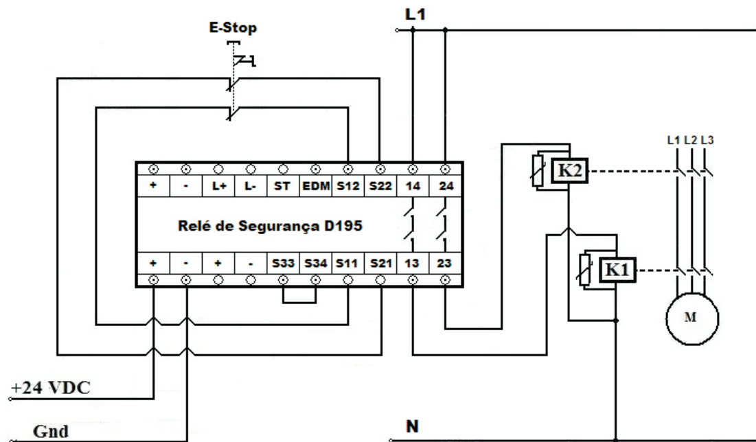
Diagrama elétrico do Relé de Segurança D195 quando utilizado como interface para o Botão de Parada de Emergência (E-Stop)
