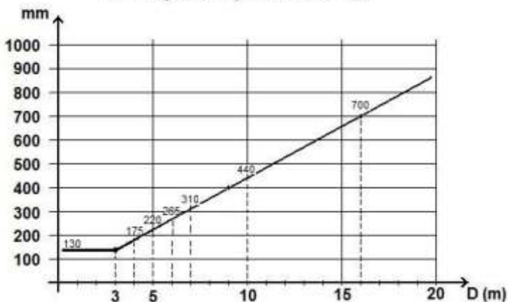
Gráfico para determinação da Distância mínima em relação às superfícies refletivas
