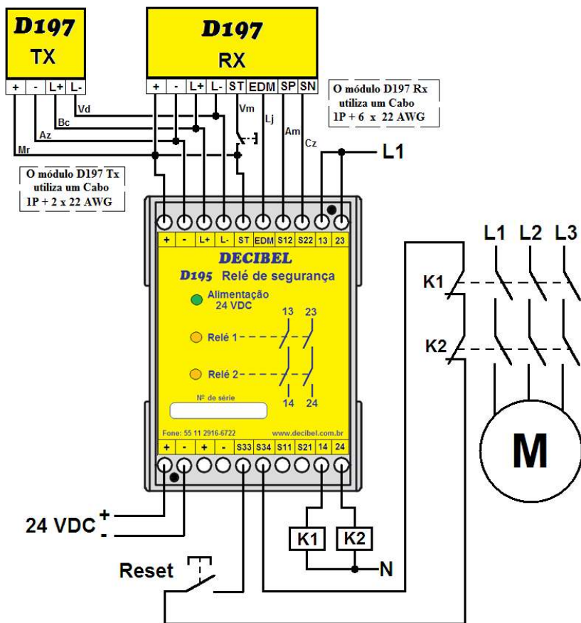
Conexão da Cortina de luz D197 com Relé de segurança D195.
