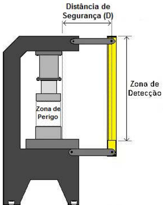
Distância de Segurança para a Zona de Perigo
