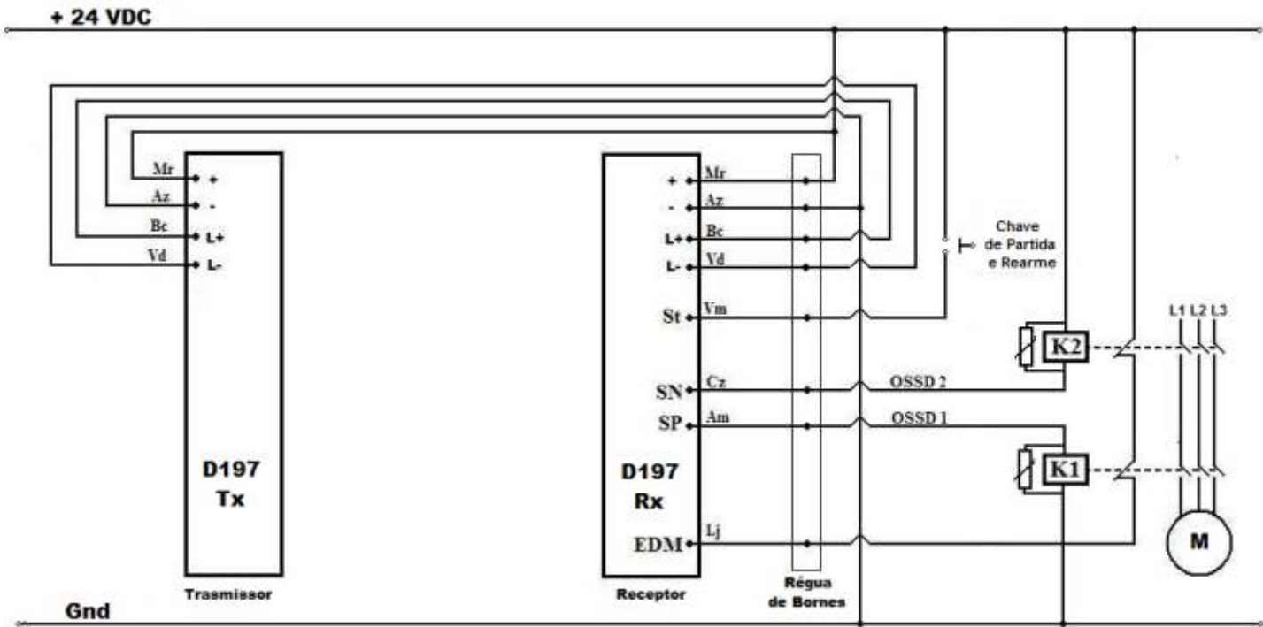
Diagrama elétrico da Cortina de luz D197 com as Contadoras
