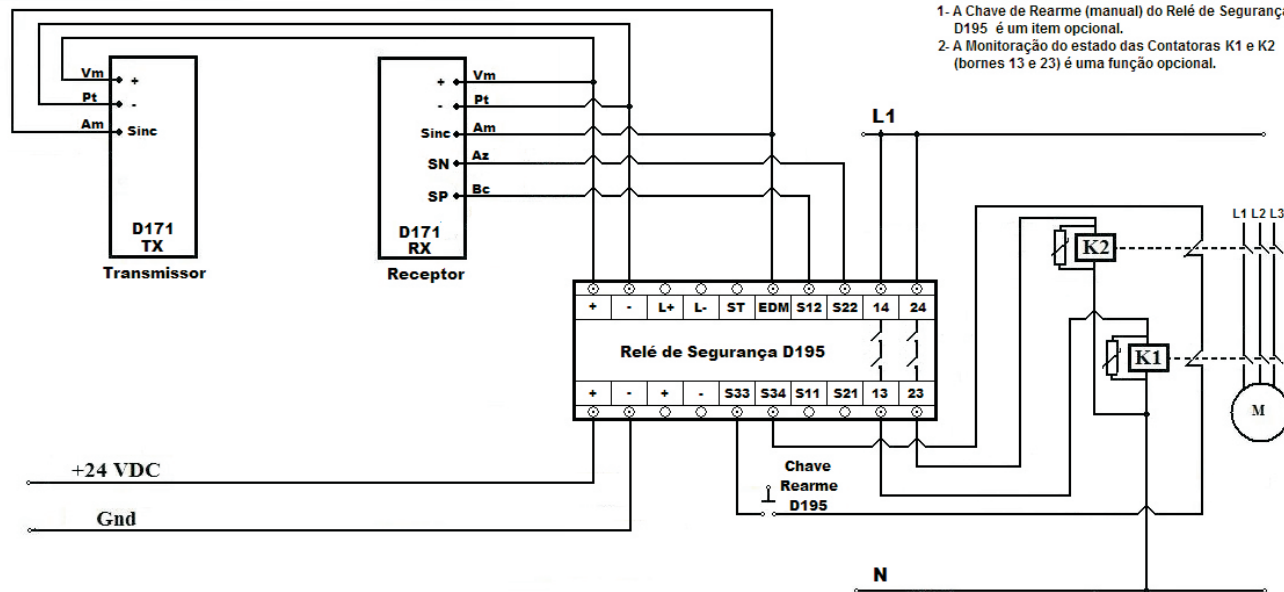
Diagrama elétrico do Relé de Segurança D195 quando utilizado como interface para o Sensor Laser D171
