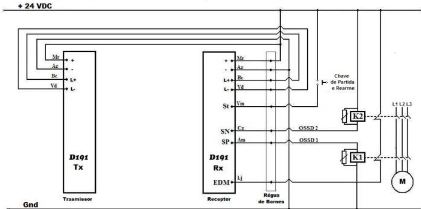
Diagrama elétrico da Barreira perimetral D191 com as contadoras
