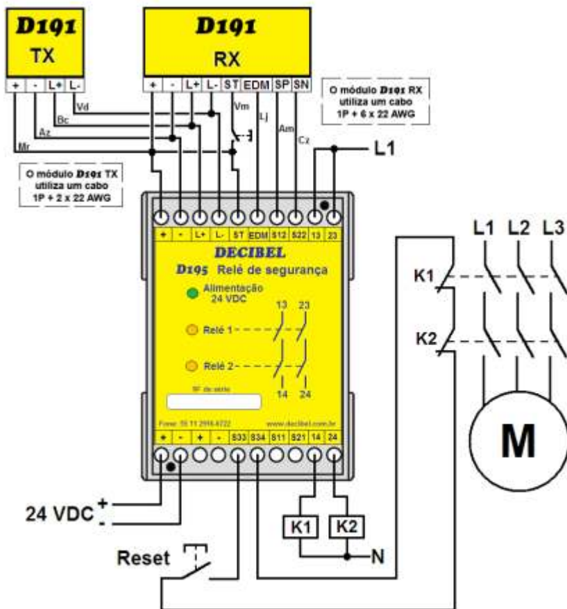
Conexão da Barreira perimetral D191 com Relé de segurança D195 .
