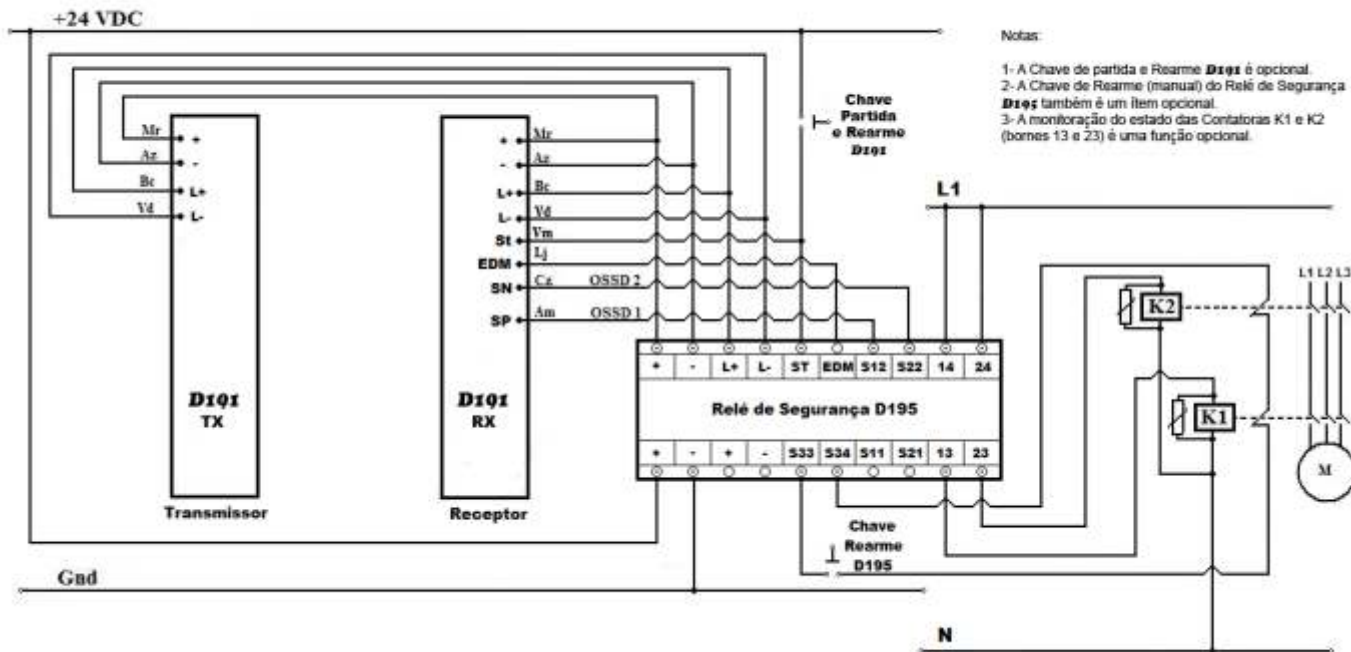
Diagrama elétrico da Barreira perimetral D191 via Relé de Segurança D195
